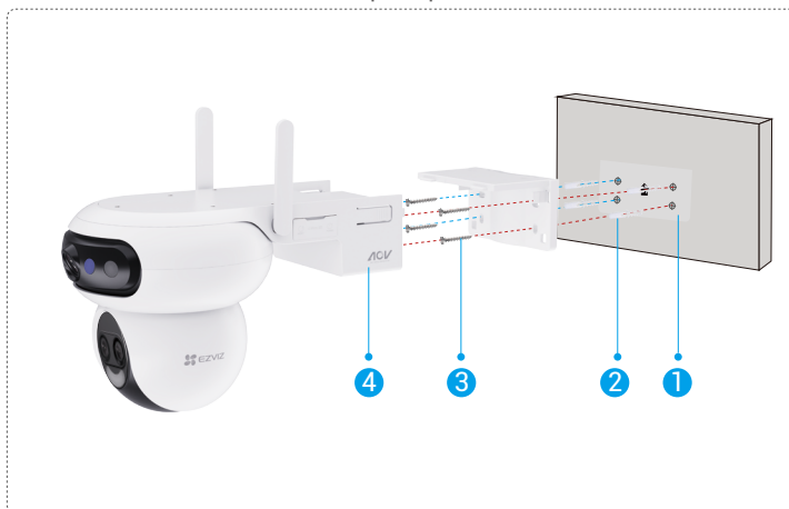
Obr. 2 Nástenné upevnenie
